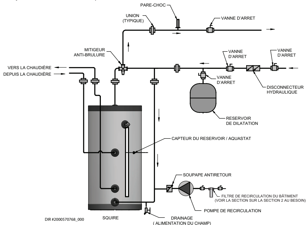
Figure 4-2 Tuyauterie d'eau domestique recommandée
